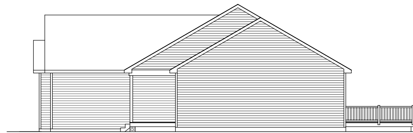
RIGHT ELEVATION
